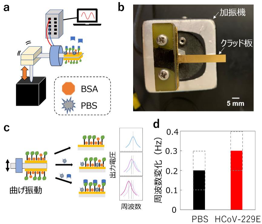
図 3 曲げ振動による HCoV-229E 検出実験
